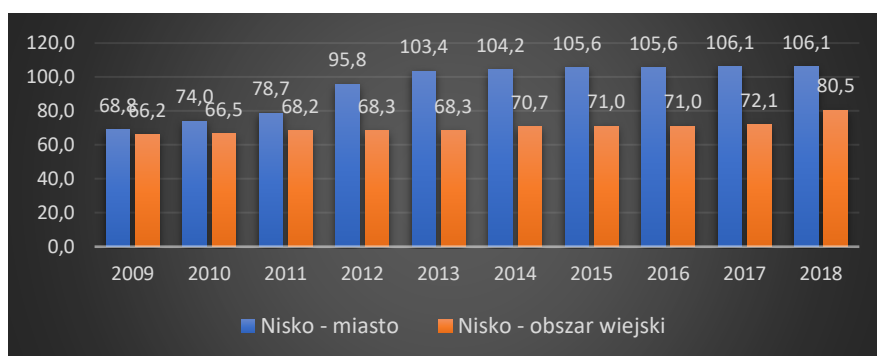
Rysunek 85 Długość czynnej sieci wodociągowej rozdzielczej w podziale na obszar
