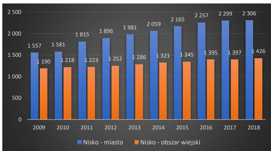
Rysunek 86 Przyłącza prowadzące do budynków mieszkalnych i zbiorowego zamieszkania w podziale na obszar
