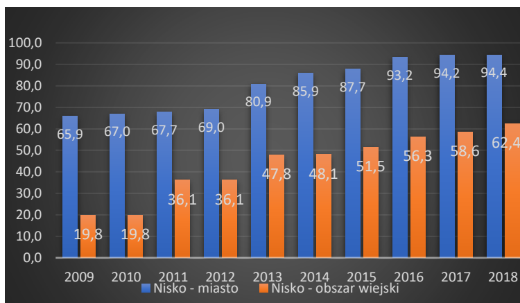
Rysunek 91 Długość czynnej sieci kanalizacyjnej w podziale na obszar
